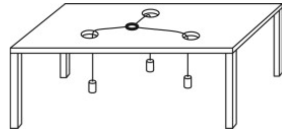
Varignon Frame
